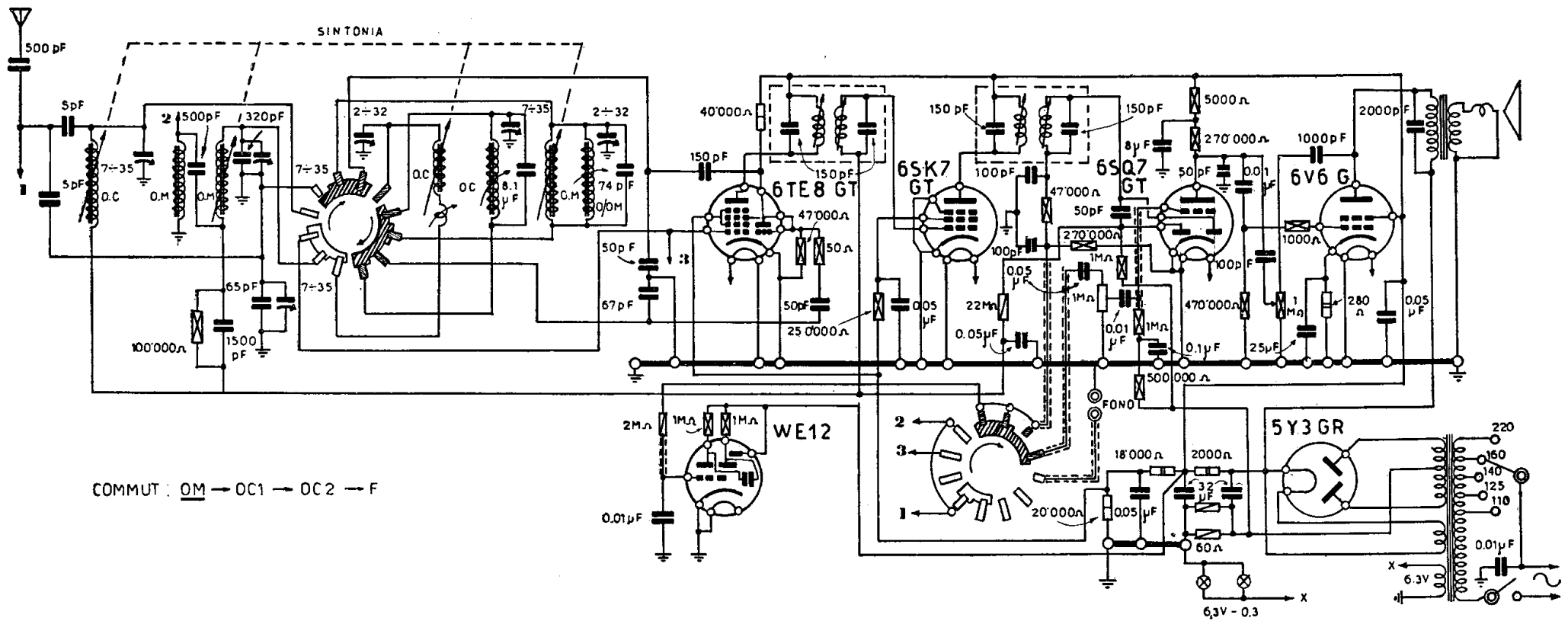
COMPAGNIA GENERALE DI ELETTRICITÀ - Mod. 395 - Medie e due corte. Commutatore in posizione medie. Media frequenza 468 kc.
